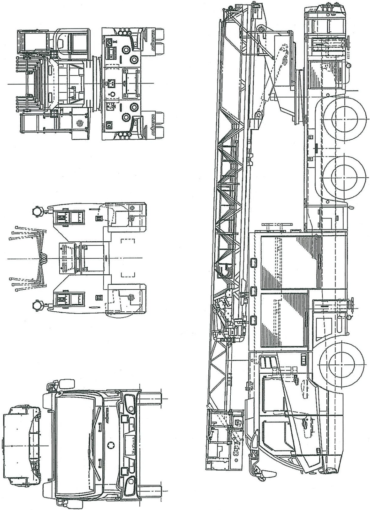
はしご付消防自動車 平面図
