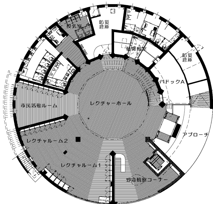
自然学習館 1階平面図
