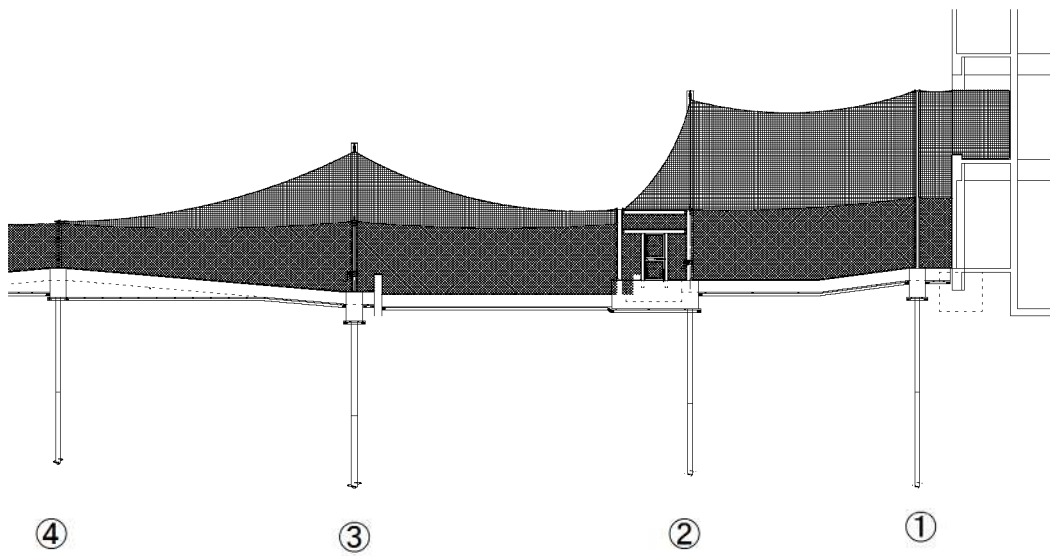
野鳥観察所 平面図・展開図
