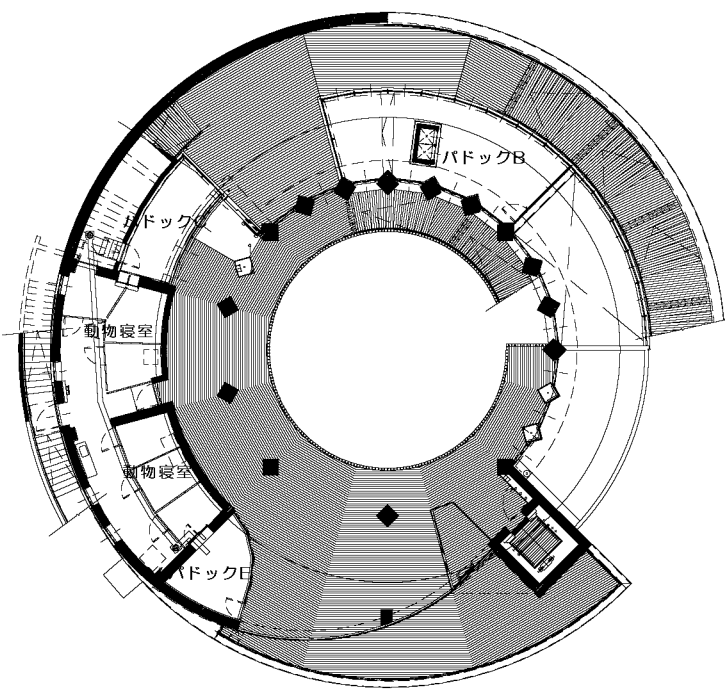
自然学習館 2階平面図
